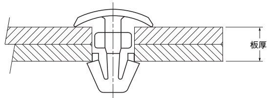
取付状態図
