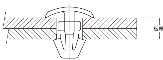
取付状態図
