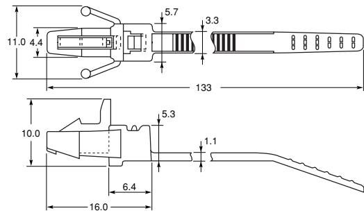
図2：リリースプッシュマウントタイ
