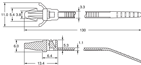
図1：プッシュマウントタイ
