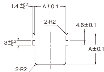
取付穴寸法図
